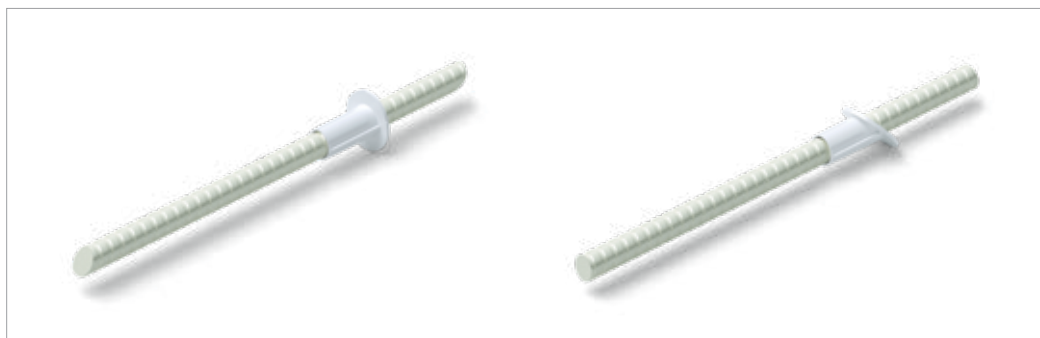
Isolink® tüüp C-SH ja C-SD koos sügavuspiirajaga viimistluseta betoonfassaadide kinnitamiseks kihtmeetodil.
